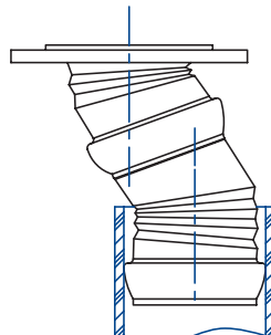
Tubería con Desfasamiento hasta 5 cm
